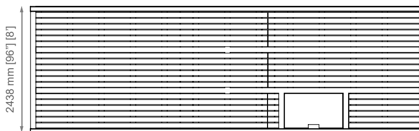
SIDE VIEW 7315 mm [288"] [24']
